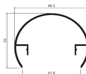
AD-1738 Anclaje Reg Superior Pasamanos red 66mm
