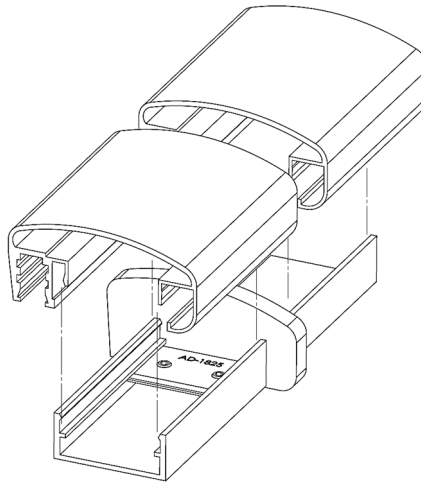
AD-1825 Unión elíptico 86x40
